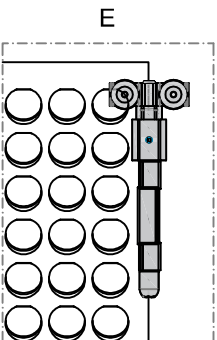
07.31.01 ÜST KAFA ARABA TOP END ROLLER
