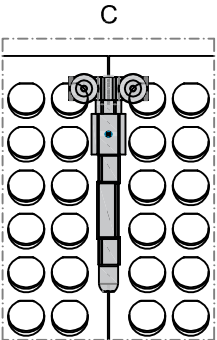
07.31.02 ÜST ORTA ARABA TOP CENTRAL ROLLER
