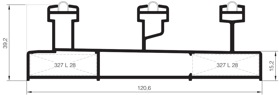
**RS83 F 03 Sineklik Kanadı için Kasa
