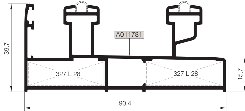
**RS83 F 03 Sineklik Kanadı için Kasa
